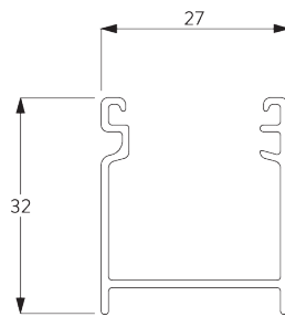
SG 10037 профиль
