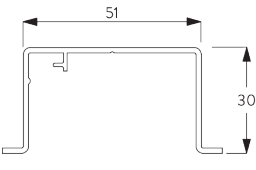
SG 11866 пазовый профиль
