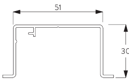
SG 11866 пазовый профиль
