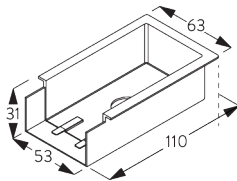
SG 11886 пазовая маска
