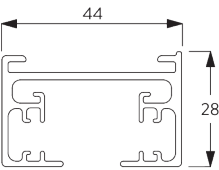
SG 11863 профиль
