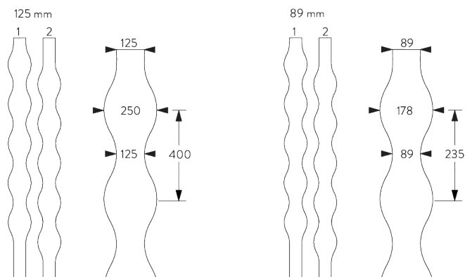
3D Vertical Waves ВОЗМОЖНО ТОЛЬКО С ЛАМЕЛЯМИ 125 мм
