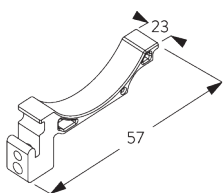
SG 2384 держатель
