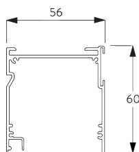
SG 2371 профиль
