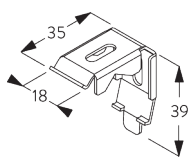
SG 2302 кронштейн
