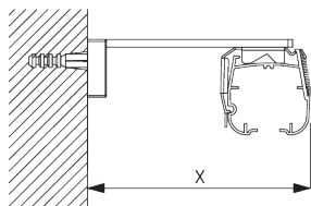
Square Smart Fix SG 11210 - SG 11215 и кронштейн SG 2302: крепеж SG 10395 (M4x6).
