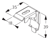
SG 2302 кронштейн
