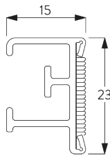
SG 2211 профиль с Velcro-лентой
