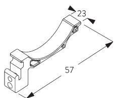
SG 2384 держатель
