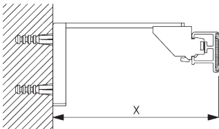
Smart Fix SG 11200 - SG 11205 и кронштейн SG 3603: крепёж SG 10492 (M4x8).
