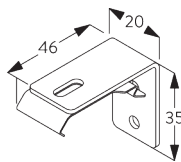
SG 2343 кронштейн 46 мм
