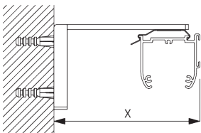
Smart Fix SG 11200 - SG 11205 и кронштейн SG 2616: крепеж SG 10395 (M4x6).
