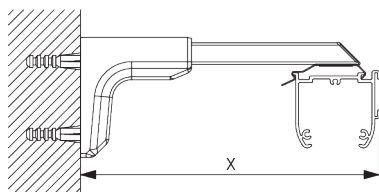
Universal Smart Fix SG 11154 - SG 11156 и кронштейн SG 2616: крепеж SG 10492 (M4x8).
