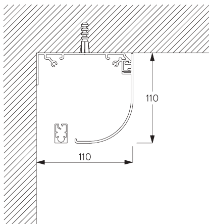
Фасция круглая
