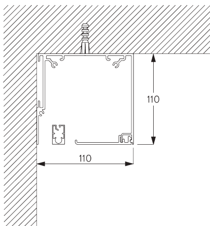
Корпус
