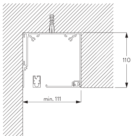
Корпус
