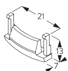
SG 11179 заглушка
