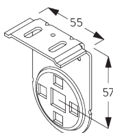
SG 11172 кронштейн
