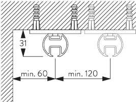
Кронштейн SG 6124
