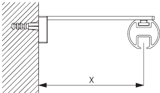
Square Smart Fix with slot SG 11216 - SG 11218: необходимо использовать крепеж SG 10492 (M4x8).
