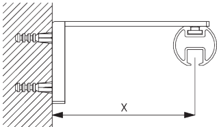
Smart Fix with slot SG 11206 - SG 11208: необходимо использовать крепеж SG 10492 (M4x8).
