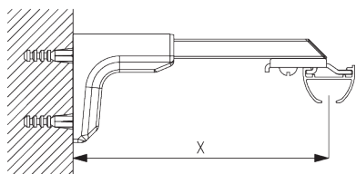
Universal Smart Fix SG 11154 - SG 11156 и кронштейн SG 3832: необходимо использовать крепеж SG 10407 (M4x10).
