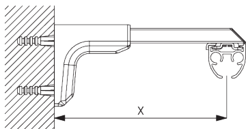
Universal Smart Fix SG 11154 - SG 11156 и монтажный зажим SG 3825: необходимо использовать крепеж SG 11158 (M4x12).
