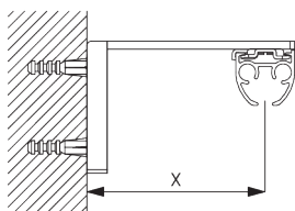
Smart Fix SG 11200 - SG 11205 и монтажный зажим SG 3825: необходимо использовать крепеж SG 10074 (M4x8).
