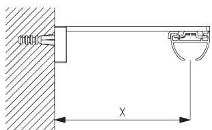
Square Smart Fix SG 11210 - SG 11215 и монтажный зажим SG 3825: необходимо использовать крепеж SG 10074 (M4x8).
