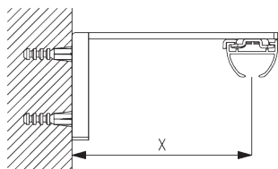
Smart Fix SG 11200 - SG 11205 и монтажный зажим SG 3825: необходимо использовать крепеж SG 10074 (M4x8).
