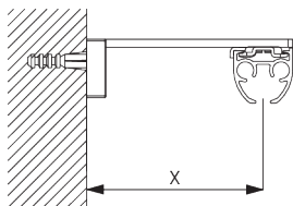
Square Smart Fix SG 11210 - SG 11215 и монтажный зажим SG 3825: необходимо использовать крепеж SG 10074 (M4x8).
