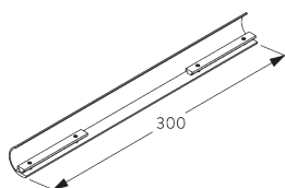
SG 6521 соединитель
