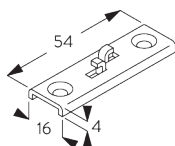
SG 6124 кронштейн
