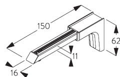
SG 11155 Universal Smart Fix 150 мм
