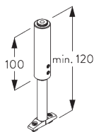
SG 6190 подвеска
