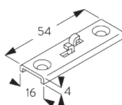
SG 6124 кронштейн
