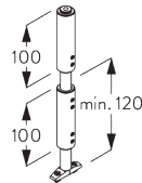
SG 6196 двойная подвеска
