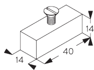
SG 6369 шпонка
