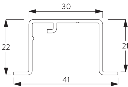
SG 11230 пазовый профиль
