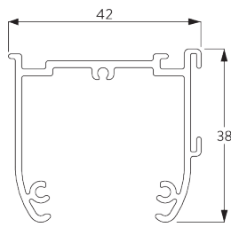
SG 2321 Profil
