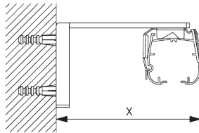
Smart Fix SG 11200 - SG 11205 und Träger SG 2302: Benötigt Schraube SG 10395 (M4x6).
