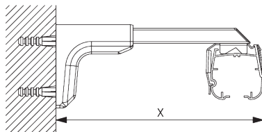
Universal Smart Fix SG 11154 - SG 11156 und Träger SG 2302: Benötigt Schraube SG 10492 (M4x8).
