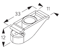
SG 2338 Drahthalter Seitenverspannung
