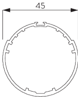
SG 2372 Rohr ø 45mm
