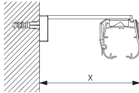
Square Smart Fix SG 11210 - SG 11215 und Träger SG 2302: Benötigt Schraube SG 10395 (M4x6).
