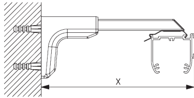
Universal Smart Fix SG 11154 - SG 11156 und Träger SG 2616: Benötigt Schraube SG 10492 (M4x8).
