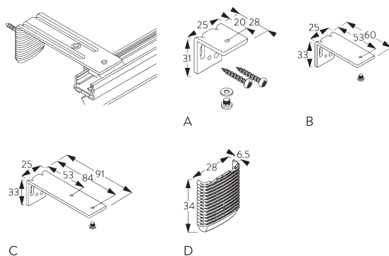
A: Tragwinkel 28 mm (M1) inkl. Schrauben
