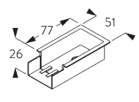
SG 10864 Nutmaske
