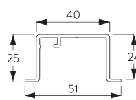
SG 10862 Nutprofil
