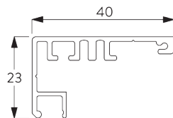
SG 11418 Seitliche Führungsschiene
