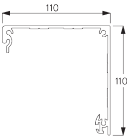
SG 10998 Kassettengehäuse 110 mm
