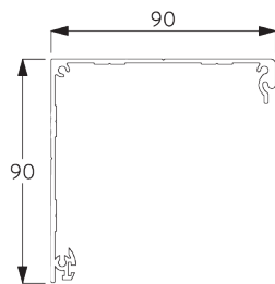
SG 10996 Kassettengehäuse 90 mm
