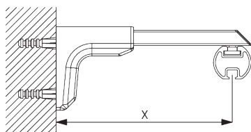
Universal Smart Fix SG 11154 - SG 11156: Benötigt Linsenschraube SG 11131 (M4x6).
