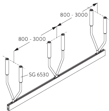
SG 6530: V-Hänger sorgen für zusätzliche Seitenstabilität.
