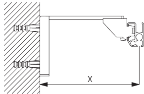
Smart Fix SG 11200 - SG 11205 und Träger SG 3603: Benötigt Schraube SG 10492 (M4x8).
