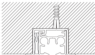
Eine Klammer SG 10157 pro Montagepunkt. Detaillierte Nutmontage siehe Silent Gliss Website.
